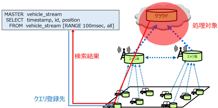
図 28 all の指定例
