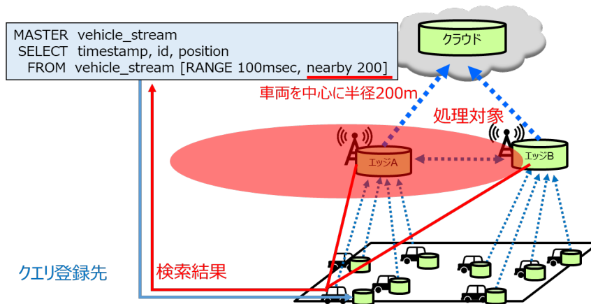
図 27 距離指定のついた nearby
