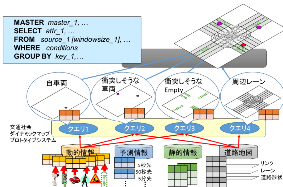
図 1 ダイナミックマップとクエリ言語
