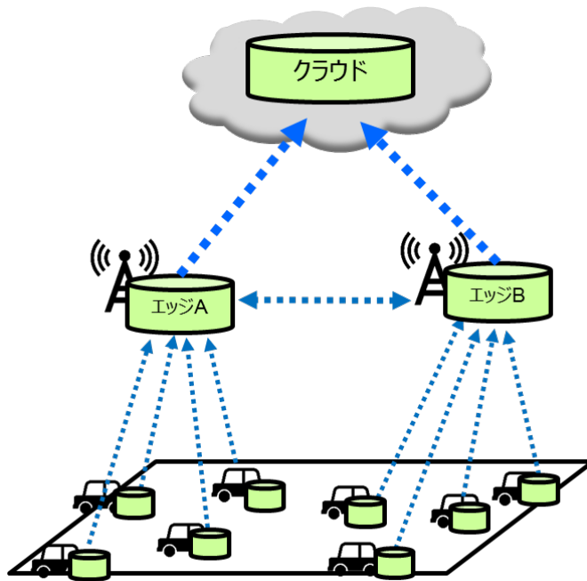
図 23 クラウド・エッジ・組込みの連携
