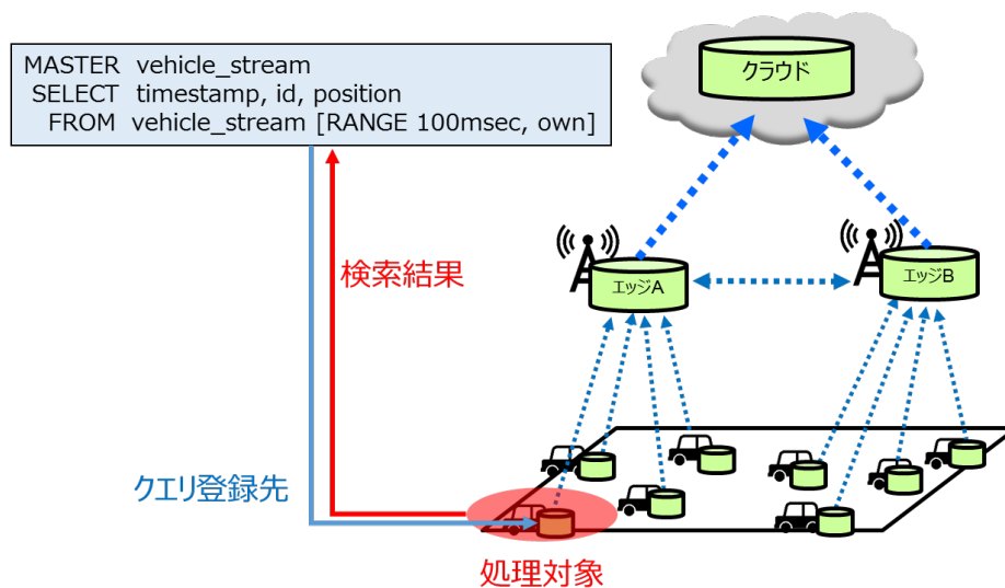
図 25 own の指定例
