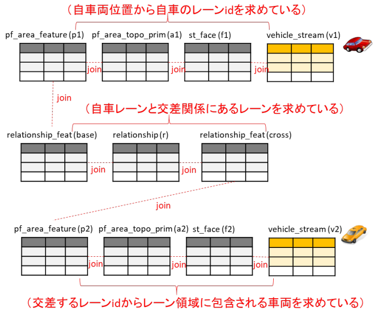
図 22 地図を介した動的情報同士の統合
